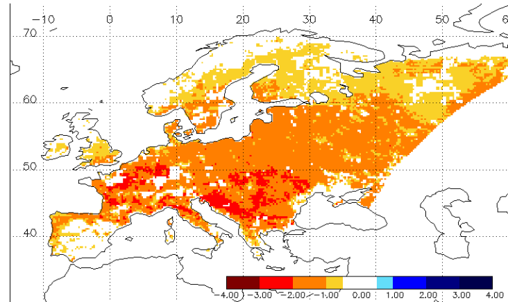
BIOME-BGC - NEE
