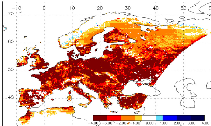
JULES-NEE
