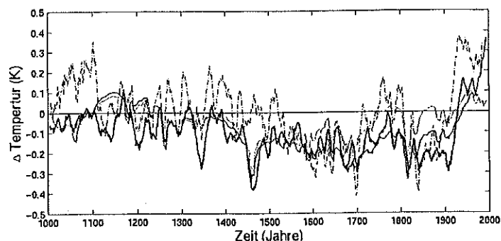
Abb. 4: Abschätzung der bodennahen Temperatur im Mittel über die Nordhemisphäre im Verlauf der letzten 1000 Jahre. Schwarze Kurve: Rekonstruktion aus Klimaarchiven (gepunktete Kurve: Jones et al. 1998; strichpunktierte Kurve: Mann et al. 1999), hellgraue Kurve: Modellrechnung mit natürlichem Antrieb (Änderung des solaren Energieflusses und Vulkanaktivität), dunkelgraue Kurve: Modellrechnung mit natürlichen und anthropogenem Antrieb (CO 2 -Emission und Landnutzung); geändert nach Bauer et al. (2003)
