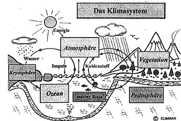
Abb. 1: Schematische Darstellung des Klimasystems und seiner Untersysteme sowie der die Untersysteme verbindenden Flüsse Fig. 1: Schematic presentation of the climate system and its subsystems including the fluxes
