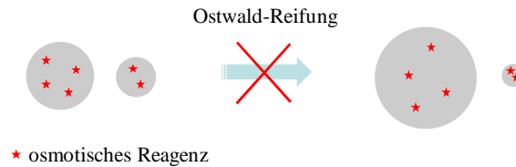
Abbildung 14: Unterdrückung der Ostwald-Reifung durch Zugabe eines osmotisch wirkenden Reagenzes.
