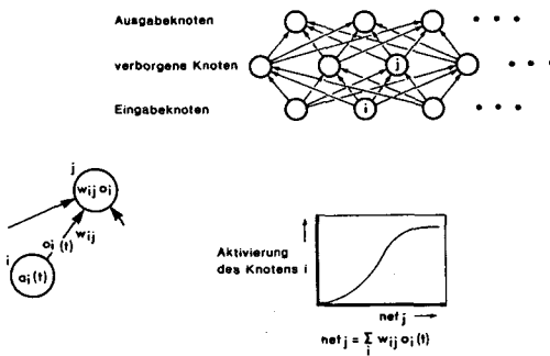
(b) Ein Netzwerk, das Wörter aus vier Buchstaben erkennt
