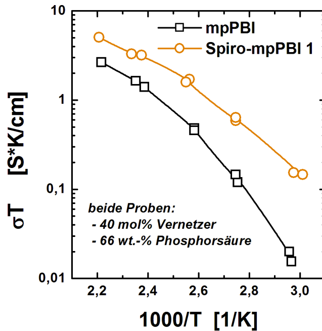
Abbildung 5.33: Arrheniusauftragung der Protonenleitfähigkeit zweier mesoporöser PBIs mit Diphenylisophthalat (mpPBI) bzw. (17) (Spiro-mpPBI-1) als lineare Comonomere. Beide Proben enthalten 40 mol.-% Vernetzer sowie 66 wt.-% Phosphorsäure; Messung bei 0% Feuchtigkeit
