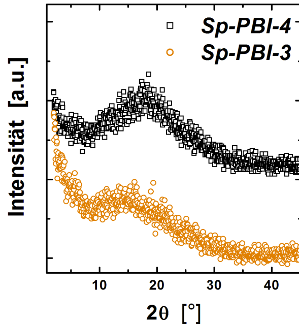
Abbildung 6.6: Weitwinkelröntgenstreuksurven der spirobifluorenbasierten PBI Netzwerke Sp-PBI-3 und Sp-PBI-4
