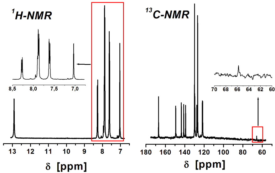
Abbildung 5.7: ^1\text{H} - sowie ^{13}\text{C} -NMR-Spektrum des Monomers (16)
