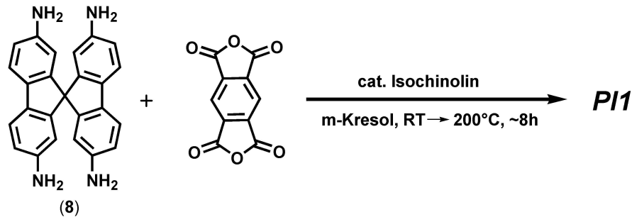
Abbildung 5.21: Syntheschema des Polyimidnetzwerks PI1
