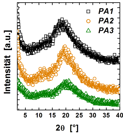
Abbildung 5.19: Weitwinkelröntgenstreuksurven der Polyamidnetzwerke PA1 - PA3; alle Proben wurden aus Aceton getrocknet
