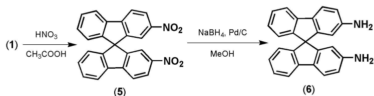
Abbildung 5.3: Syntheseroute zum 2,2'-Diamino-9,9'-Spirobifluoren (6)
