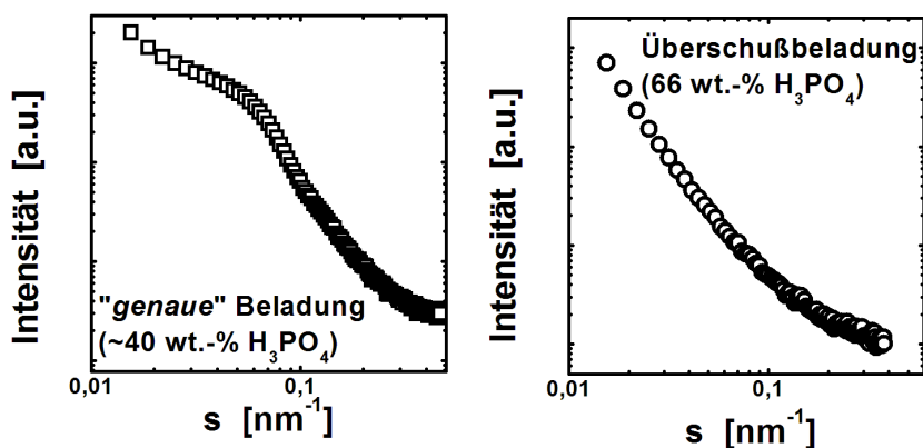
Abbildung 4.14: SAXS-Kurven der genau beladenen Probe (links) und der überschußbeladenen Probe (rechts)
