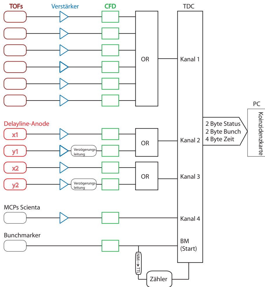
Abbildung 3.14: Schema der Signalführung für Elektron-Elektron-Koinzidenzmessungen an einem Synchrotron. Während es im Single-Bunch-Modus ausreichend ist, alle Signale bezüglich des Bunchmarkers zu messen, muss im Multi-Bunch-Modus die Zeitkorrelation zwischen zwei Elektronen ausgenutzt werden. Deshalb wird zusätzlich die genaue Eintreffzeit eines Elektrons im Scienta registriert. Die Verzögerungsleitungen sind notwendig, um auch nach der Veroderung die jeweils beiden Enden der Delayline eindeutig zuzuordnen zu können.
