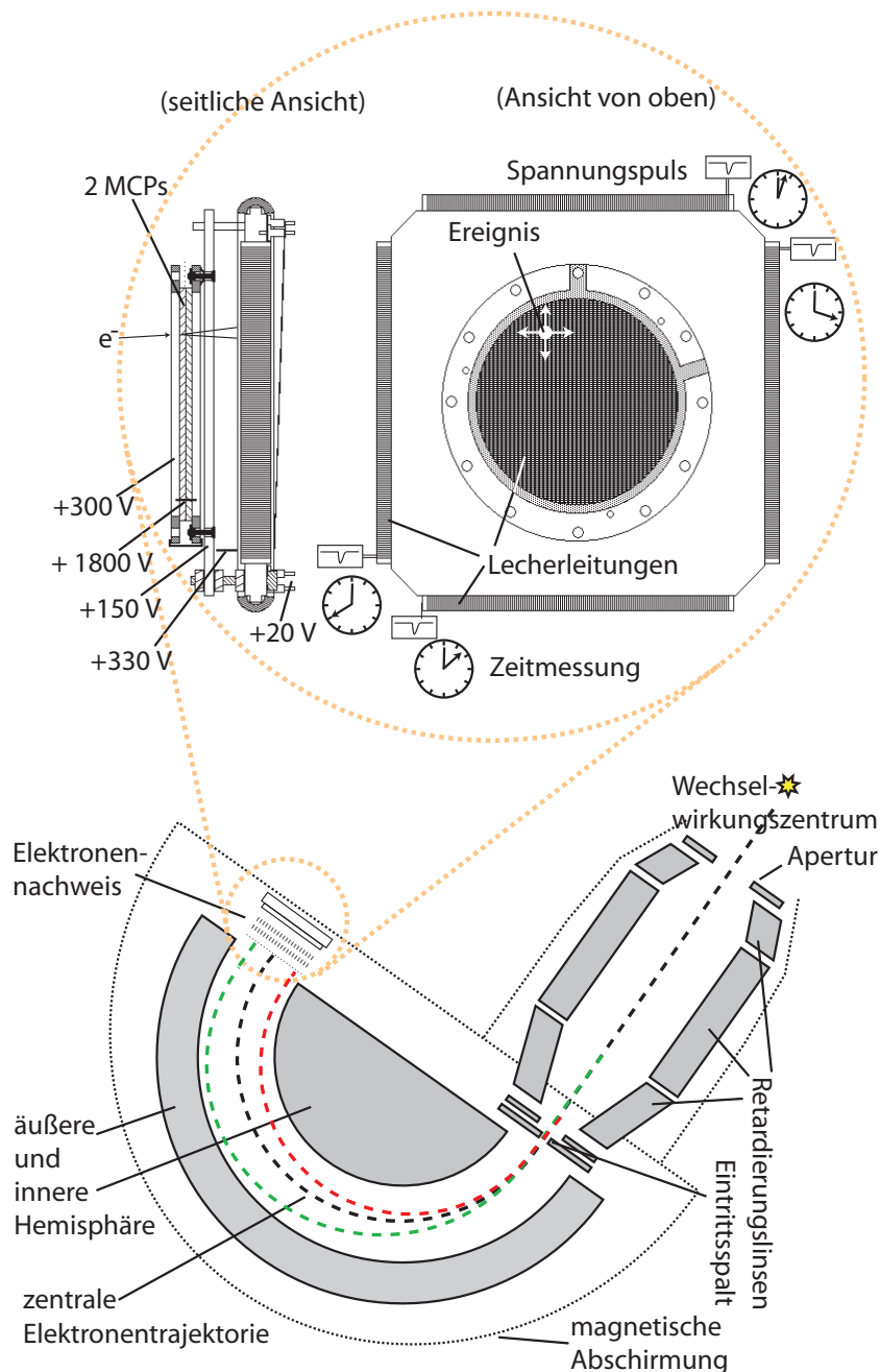
Abbildung 3.13: Im unteren Teil der Zeichnung ist der Analysator (Scienta ES200) mit den wichtigsten elektronenoptischen Elementen im Querschnitt dargestellt. Zur Verdeutlichung des dispersiven Effektes sind außerdem die Flugbahnen von senkrecht einfallenden Elektronen eingezeichnet, die im Analysator eine kinetische Energie größer (grün), gleich (schwarz) oder kleiner (rot) der Passenergie haben. Für den schnellen Elektronennachweis ist der hemisphärische Elektronenanalysator mit einer Delayline-Anode (im orangenen Kreis) ausgerüstet worden. Nach dem Auftreffen eines Elektrons tritt aus der Rückseite der MCPs eine Elektronenwolke, trifft auf einen kleinen Bereich der Lecherleitungen und erzeugt in alle vier Richtungen laufende elektrische Pulse.
