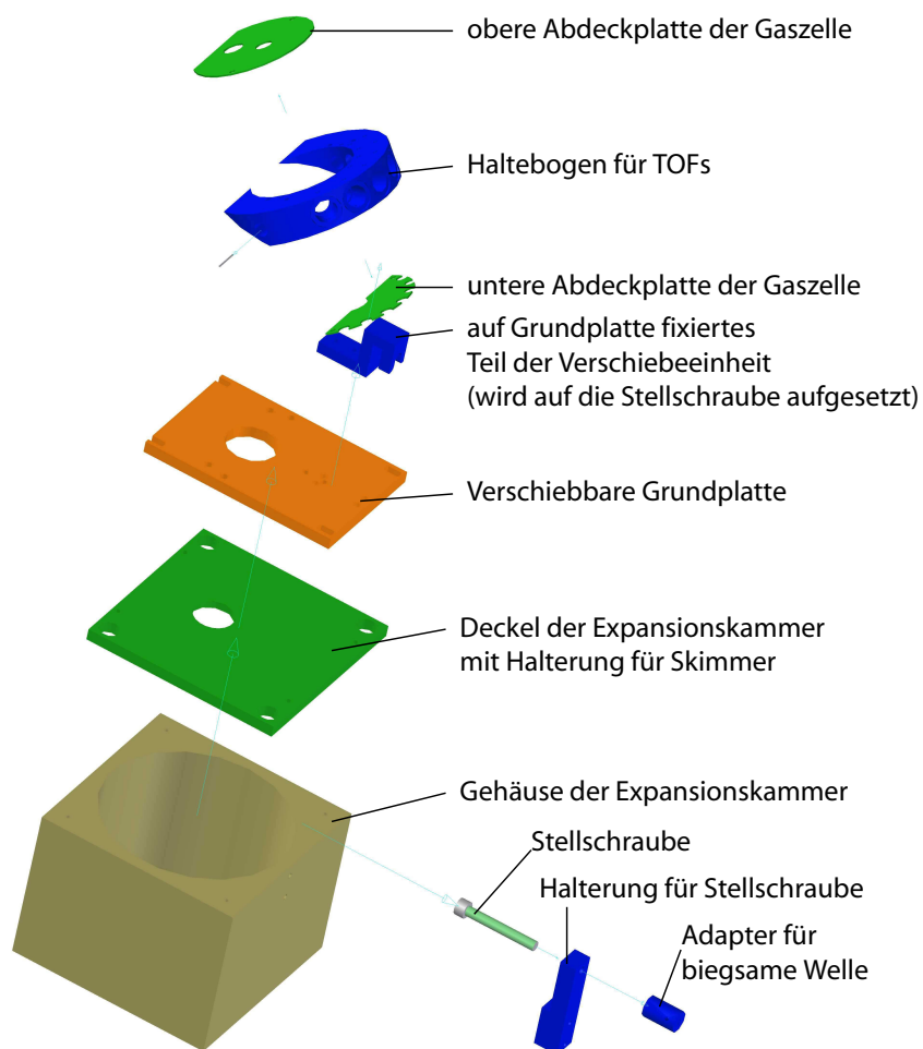
Abbildung 9.1: Explosionsdarstellung des oberen Teils der Expansionskammer.
