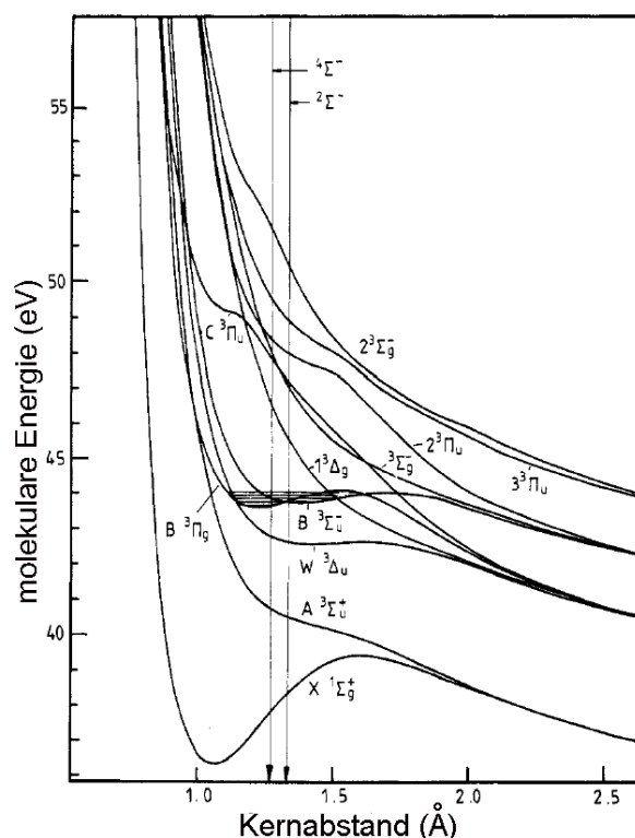
Abbildung 6.3: Berechnete Potenzialkurven für \text{O}_2^{2+} aus [160]. Die senkrechten Pfeile zeigen die Franck-Condon-Zonen des Dublett- und des Quartett-Zustands an.
