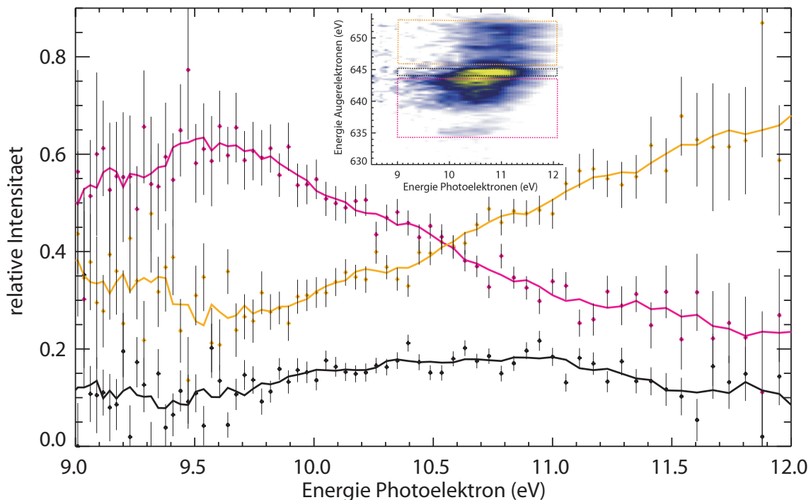
Abbildung 5.4: Relativer Beitrag zum gesamten Auger-Spektrum in Abhängigkeit von der Energie des koinzidenten Photoelektrons. A4 (schwarz), A5 + A6 + A7 (magenta), A1 + A2 + A3 (orange).
