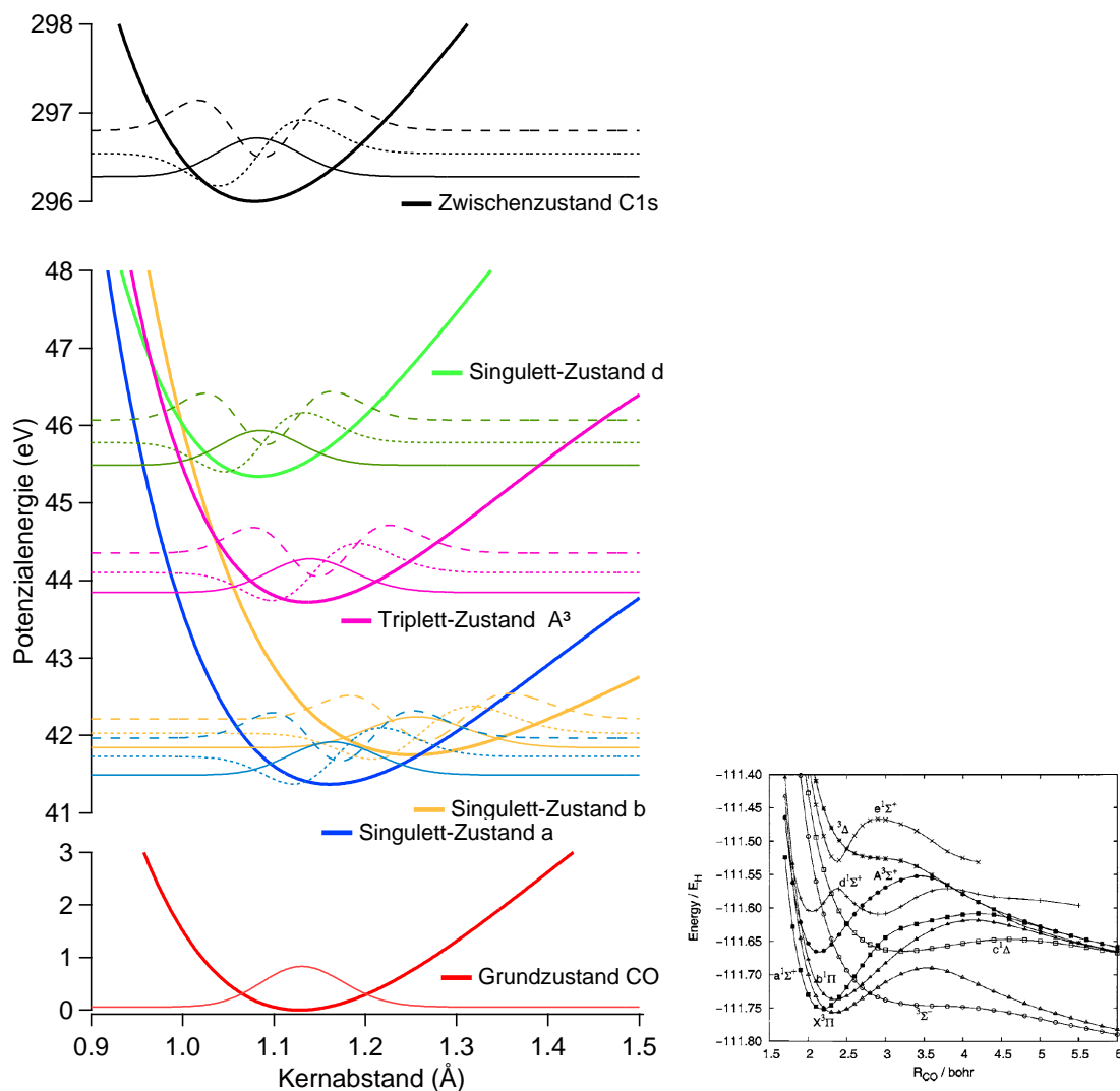
Abbildung 4.1: Berechnete Potenzialkurven und Wellenfunktionen von CO, CO + und CO ++ . Der Übersichtlichkeit halber sind jeweils nur die ersten drei Vibrationszustände eingezeichnet. Im kleinen Bild sind die theoretischen Potenzialkurven aus Referenz [126] über Bohrschem Radius ( r_{bohr} = 0,53 \text{ \AA} ) und Hartree-Energie ( 1E_H = 27,2 \text{ eV} ) aufgetragen.
