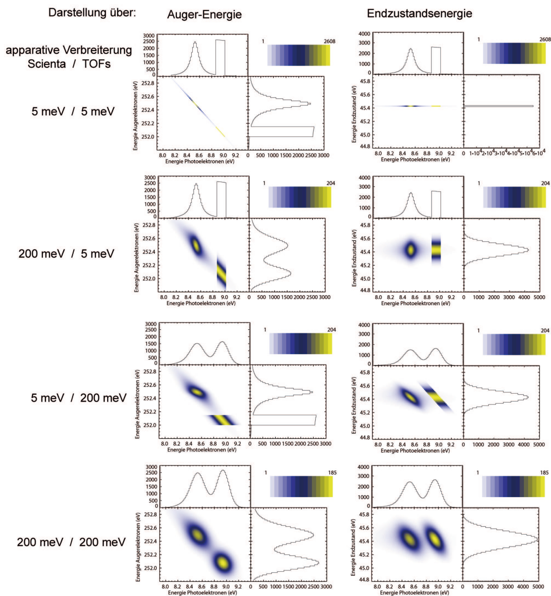
Abbildung 4.6: Simulation der Auswirkung der apparativen Energieverbreiterung auf das Erscheinungsbild der Koinzidenzstrukturen. Auf der linken Seite ist jeweils ein Koinzidenzspektrum über der Energie der Auger- und Photoelektronen dargestellt, rechts dasselbe Spektrum transformiert zu einer Darstellung mit der Endzustandsenergie als Ordinate (und der Photoelektronenenergie als Abszisse). Für die Simulation wurden zwei Lorentzlinien mit jeweils 150 meV Breite verwendet, wobei die eine Linie entlang der Photoelektronenenergie durch eine Rechteckfunktion ersetzt wurde. Die als gaußförmig angenommene apparative Verbreiterung der Detektoren variiert von oben nach unten. Man erkennt deutlich, wie stark die Lage der Koinzidenzstrukturen vom Auflösungsvermögen der Elektronendetektoren beeinflusst wird. Die Intensitätsskalierungen sind willkürlich gewählt.
