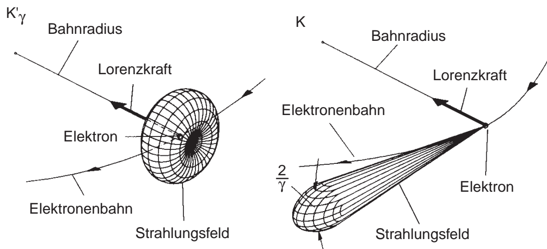
Abbildung 3.1: Abstrahlverhalten eines relativistisch schnellen Elektrons im mitbewegten Bezugssystem (links) und im Laborsystem (rechts) (aus [97]).
