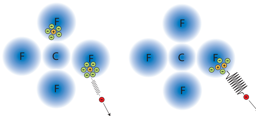
Abbildung 5.5: Aufgrund der Polarisationsabschirmung der Lochzustände (orange) durch Elektronen (grün) kann es je nach Endzustandskonfiguration zu einer unterschiedlichen Coulomb-Kraft (als Feder symbolisiert) auf ein emittiertes Photoelektron (rot) kommen. Verteilen sich beide Löcher auf zwei Fluoratome (links), dann ist diese Anziehung schwächer als im Falle einer Lokalisation beider Löcher im gleichen Fluoratom (rechts).
