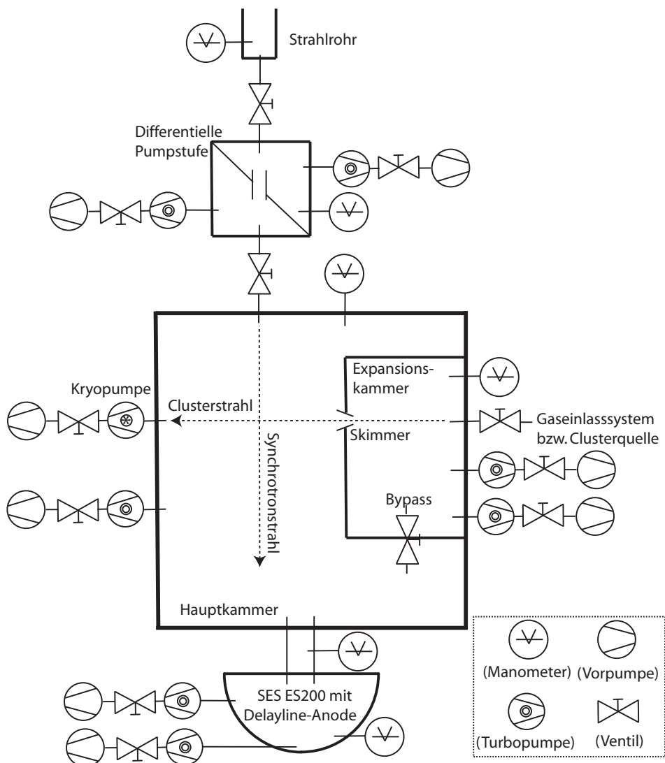
Abbildung 3.5: Schema der Vakuumerzeugung und -messung in den verschiedenen Rezipienten.
