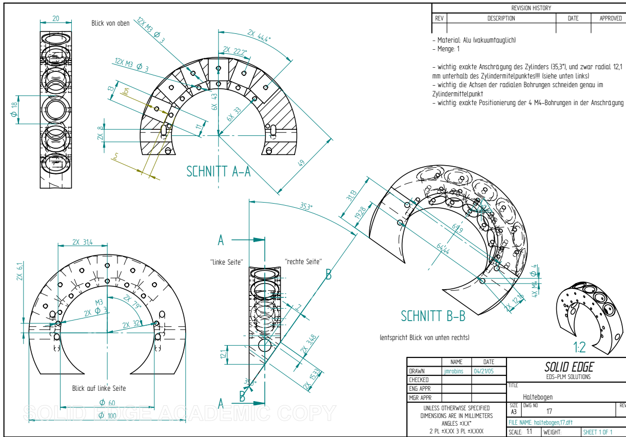
Abbildung 9.3: Technische Zeichnung des Haltebogens, mit dem die TOFs an der Expansionskammer fixiert werden.
