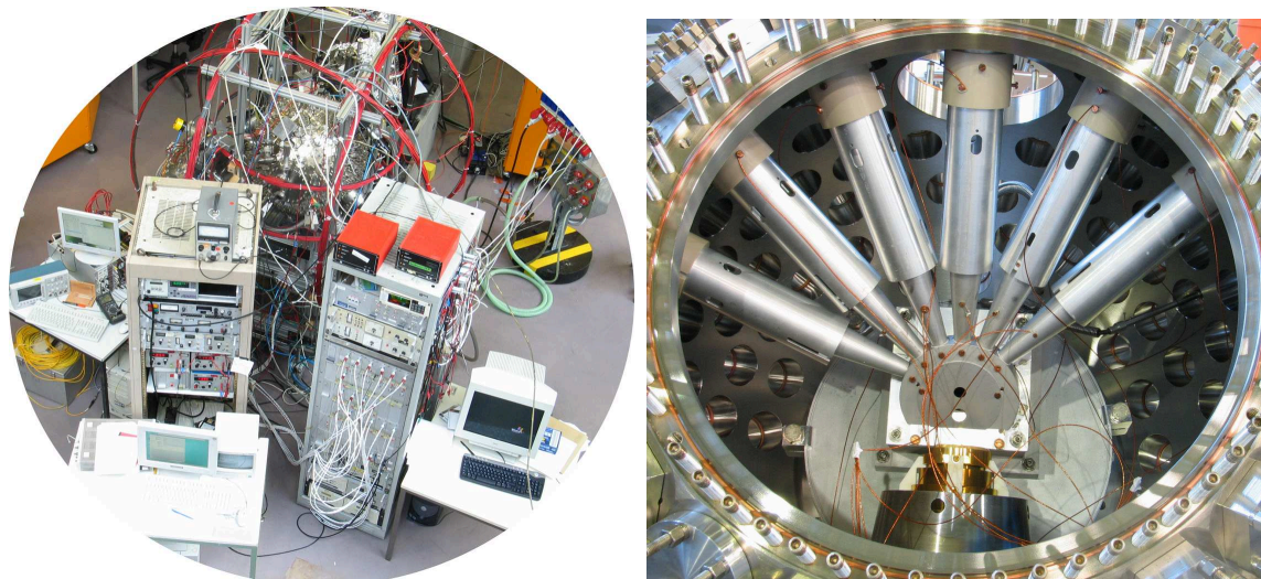
Abbildung 3.6: Linkes Bild: Die Vakuummehrung (von roten Spulen umgeben) ist an das Strahlrohr angeschlossen. Außerdem sind verschiedene Peripheriegeräte wie Messrechner, Pumpensteuerungen, Strom- und Spannungsversorgungen zu erkennen. Rechtes Bild: Die sechs TOFs eingebaut in die Vakuummehrung. Ein in Richtung TOF fliegendes Elektron durchläuft also erst 30 mm feldfreie Gaszelle, bevor es ab der 4 mm dicken konisch geweiteten Blende das vordere Retardierungspotenzial spürt. Nach 110 mm in der konischen Retardierungsröhre kommen weitere 85 mm hintere Retardierungsstrecke sowie 3 mm Beschleunigungsstrecke zum MCP hinzu.
