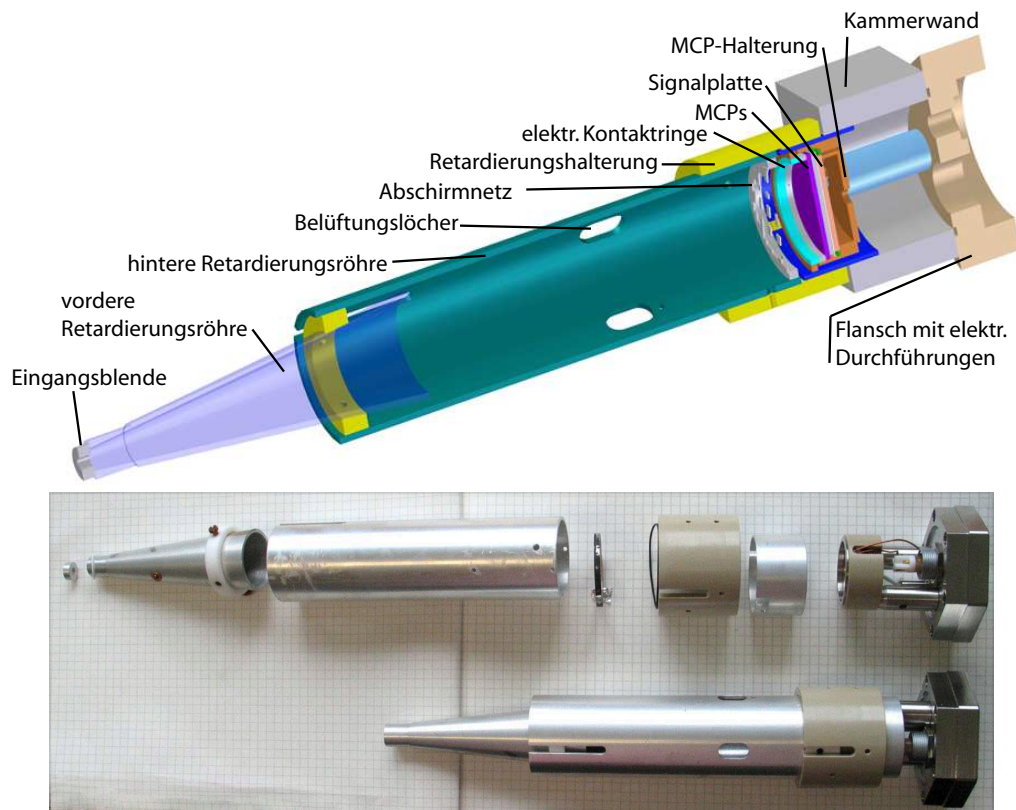
Abbildung 3.7: Oben: Geschnittene Ansicht eines TOF-Spektrometers. Unten: TOF-Spektrometer in seine Einzelteile zerlegt.
