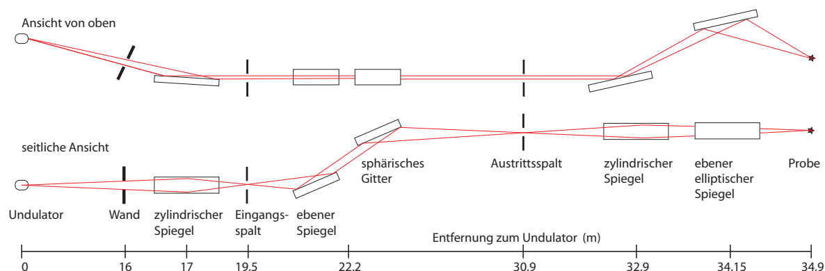
Abbildung 3.4: Strahlengang im Strahlrohr UE52-SGM. Hinter dem Beugungsgitter mit 900, 1200 oder 1500 l/mm breiten sich die spektralen Anteile des Lichts in verschiedene Richtungen aus. Im Zusammenspiel mit dem Undulator wird nun der Monochromator so eingestellt, dass das Maximum der Undulatorstrahlung den Austrittsspalt trifft. Durch das Verkleinern dieses Spaltes kann die Monochromasie im Wechselwirkungszentrum weiter erhöht werden.
