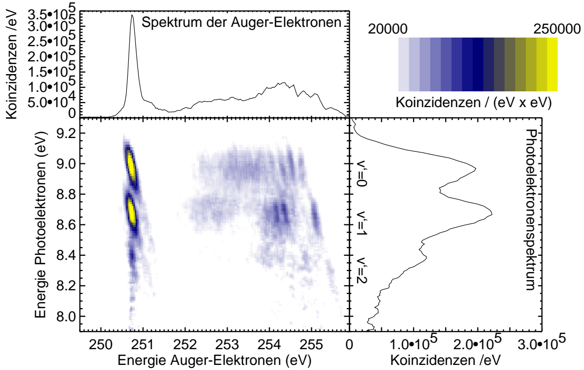
Abbildung 4.3: Zweidimensionales Koinzidenzspektrum von Kohlenmonoxid nach C1s -Photoionisation mit 305 eV und nachfolgendem KVV -Auger-Zerfall. Rechts ist die Summe aller koinzidenten Photoelektronen abgebildet, oben das Histogramm der Auger-Elektronen. In der farbkodierten Karte selbst sind die physikalisch korrelierten Elektronenpaare normiert auf Energieeinheiten eingetragen.
