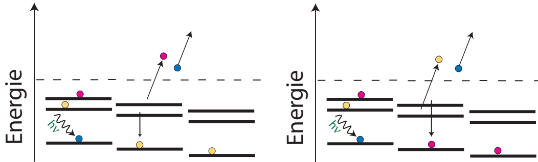
Abbildung 2.3: Schema des Auger-Zerfalls. Der normale Auger-Zerfall wird in einen direkten Prozess (links) und einen sogenannten Austauschprozess (rechts) unterteilt [33]. Aufgrund der jeweils gleichen Energie des Auger-Elektrons (links pink und rechts gelb gezeichnet) sind beide Prozesse experimentell voneinander nicht zu unterscheiden.
