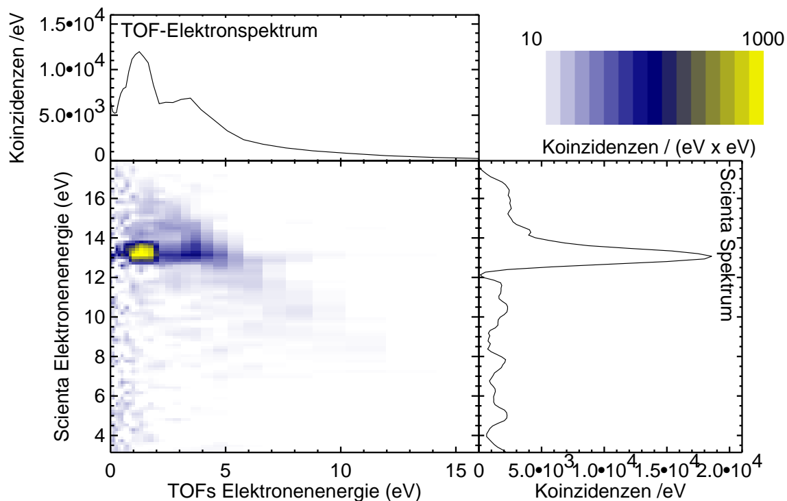
Abbildung 7.1: Elektron-Elektron-Koinzidenzspektrum von Neonclustern bei Bestrahlung mit 61 eV Photonenenergie.
