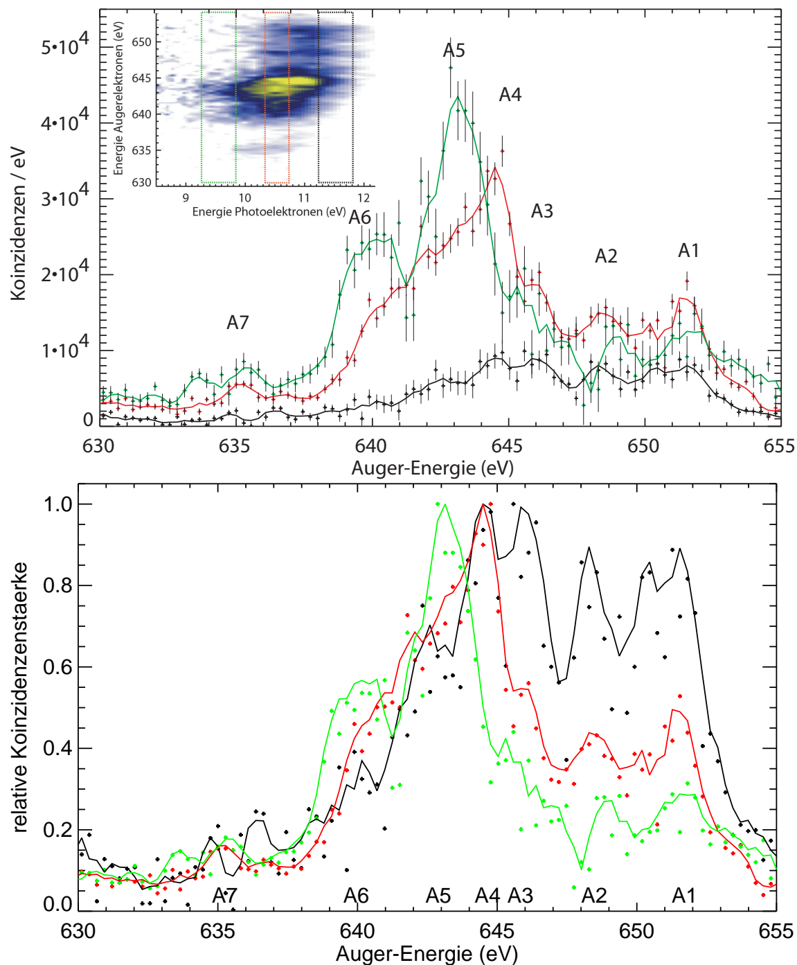
Abbildung 5.3: Das Fluor- KVV -Auger-Spektrum von \text{CF}_4 bei verschiedenen Energien des Zwischenzustandes. Dargestellt ist jeweils das Auger-Spektrum koinzident mit schnellen (schwarz), moderaten (rot) und langsamen (grün) Photoelektronen, durch die farbigen Bereiche in der eingesetzten Koinzidenzkarte markiert. Um die Spektren besser miteinander vergleichen zu können, sind sie im unteren Bild auf selbe Höhe normiert worden.
