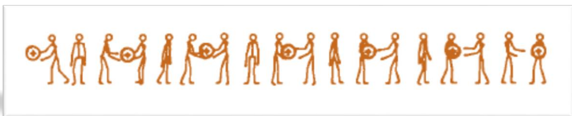
Abb. 1.3: Modell des Grotthuss -Mechanismus; die Protonen werden entlang Wasserstoffbrücken weitergereicht. [18]
