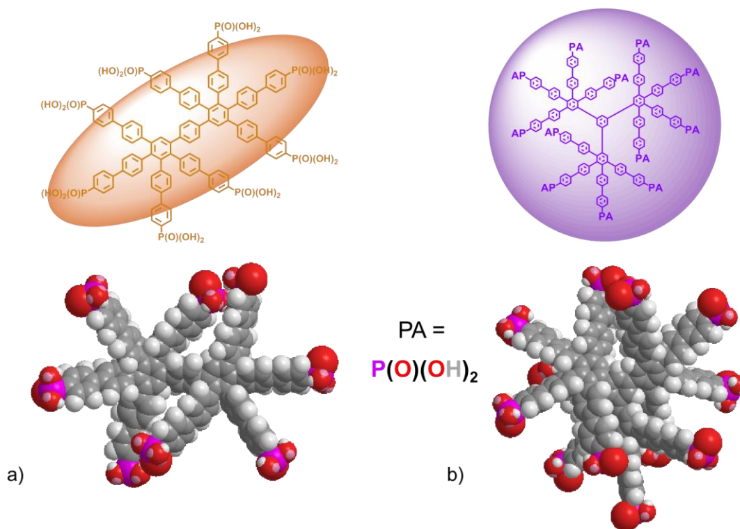
Abb. 3.36: 3D-Karlotenmodelle der Dendrimere a) 3-42 und b) 3-43 , berechnet über ChemDraw 3D mit MMFF94 Energieminimierung für die Gasphase.
