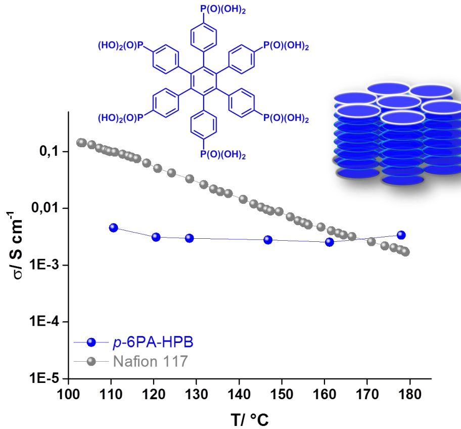
Abb. 1.7: Schematische Darstellung der hexagonalen, kolumnaren Selbstorganisation in p -6PA-HPB sowie die korrespondierenden Protonenleitfähigkeitsplots vs. Temperatur unter 1 bar Wasserdampf-atmosphäre für p -6PA-HPB (●) und Nafion ® 117 (●).
