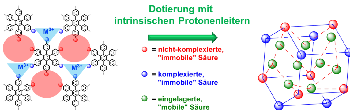
Abb. 2.4: Idealisiertes Strukturmodell eines dotierten, nicht-klassischen Aluminiumphosphonat-Netzwerkes mit p -6PA-HPB als Linker und einem dreiwertigen Metallkation als Konnektor.
