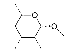
\alpha -glycosidic bond
