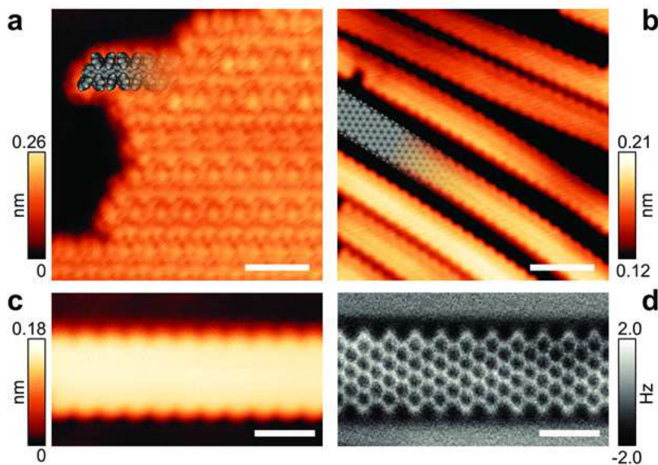
Abbildung 49: (a) STM Topografie Bild und strukturelles Modell des Polymerintermediats 1-PP1 . (b) STM Topografie Bild und strukturelles Modell des GNRs 1-GNR1 . (c) Hochaufgelöstes STM Topografie Bild eines einzelnen 9-AGNR . (d) Hochaufgelöstes nc-AFM Frequenzverschiebungsbild von 9-AGNR mit einer CO-funktionalisierten AFM-Spitze
