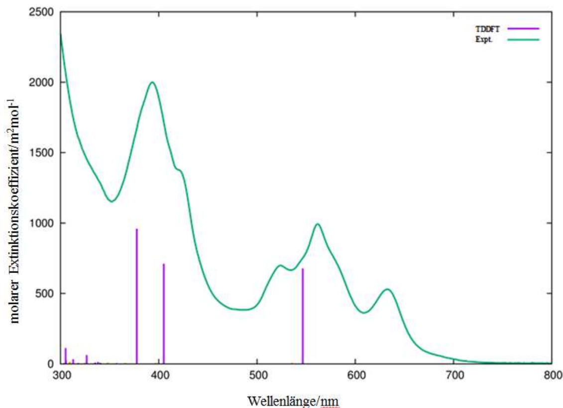
Abbildung 151: UV/Vis-Spektrum von 1-113 gemessen in THF (türkis) und TDDFT-Berechnungen der vertikalen Übergänge (magenta)
