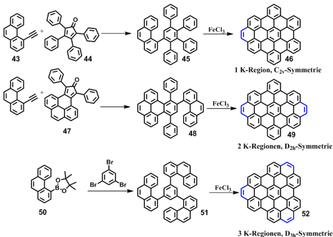
Abbildung 36: Synthese von HBC-Derivaten mit 1-3 K-Regionen
