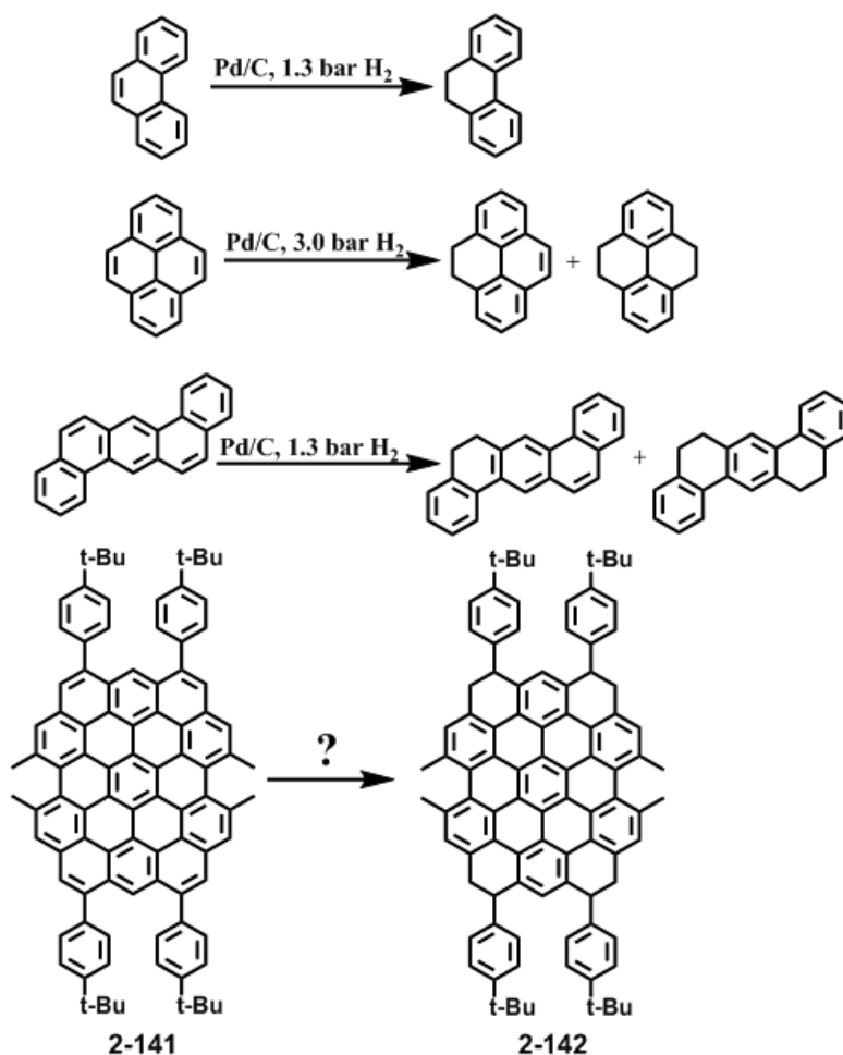
Abbildung 171: Katalytische Hydrierung von K-Regionen an PAHs
