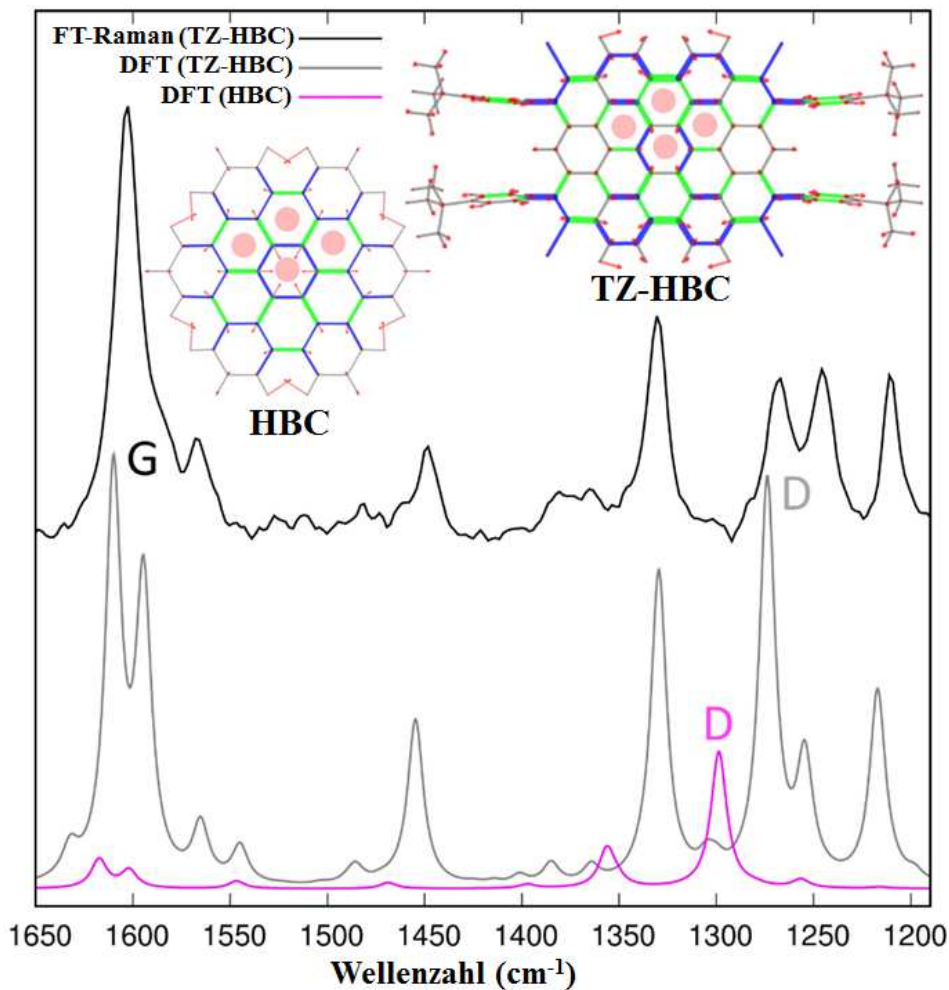
Abbildung 147: Raman-Spektrum von 1-113
