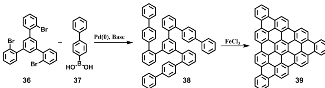
Abbildung 28: Synthese von C60 via Suzuki-Kupplung
