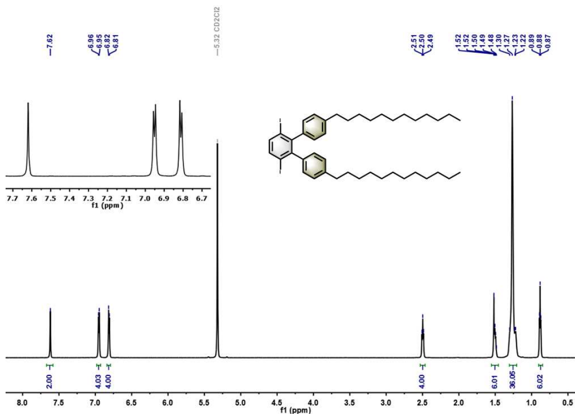
Abbildung 71: ^1\text{H-NMR} -Spektrum von 1-23 gemessen in \text{C}_2\text{D}_2\text{Cl}_4 bei RT
