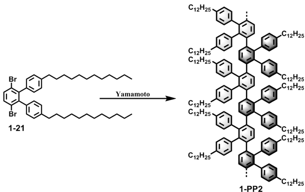
Abbildung 69: Yamamoto-Polymerisation von Monomer 1-21
