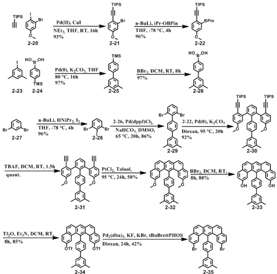
Abbildung 99: Syntheseroute zum U-förmigen Monomer 2-35 ohne externen Phenylrest
