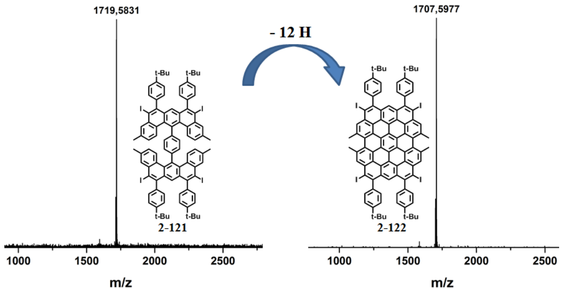
Abbildung 160: MALDI-ToF-MS-Analyse der Cyclodehydrierung von 2-121 zu 2-122
