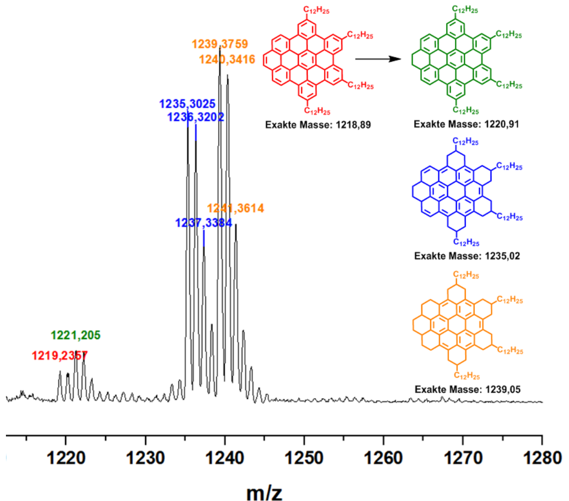
Abbildung 173: MALDI-ToF-Spektrum nach der Hydrierung von HBC mit einer K-Region mit Rh/C als Katalysator bei einem H_2 -Druck von 60 bar gemessen mit TCNQ als Matrix
