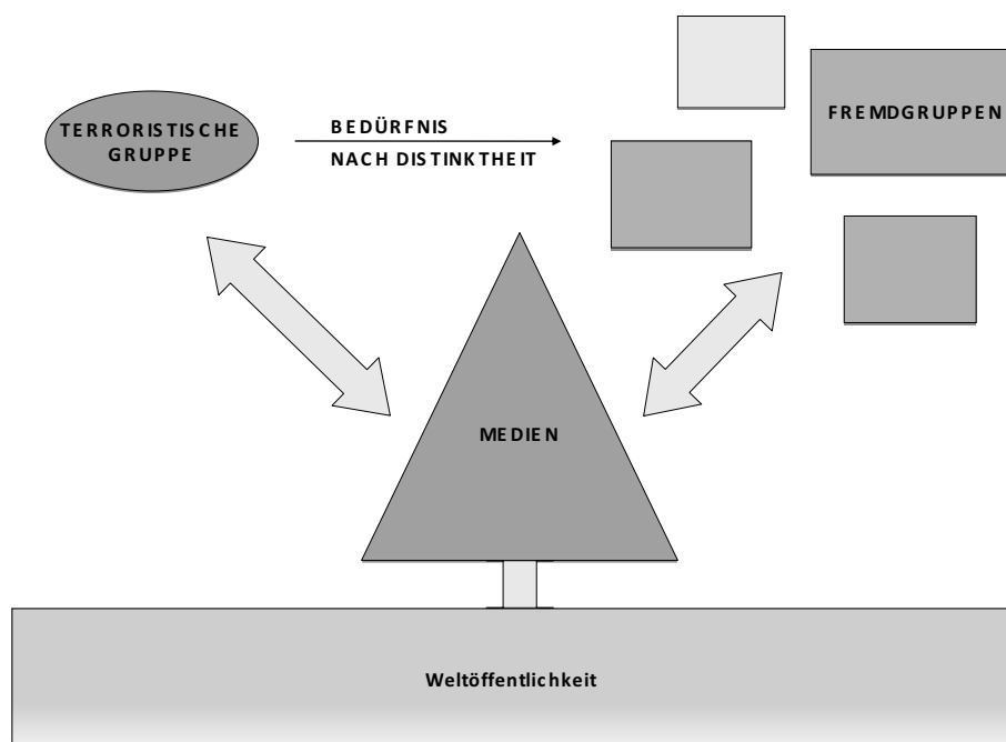
Abbildung 5: Bedürfnis nach Abgrenzung bei gleichzeitiger sozialer Abhängigkeit.
