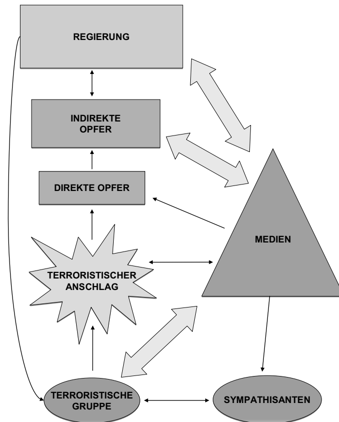
Abbildung 1: Funktionsweise des Terrorismus.
