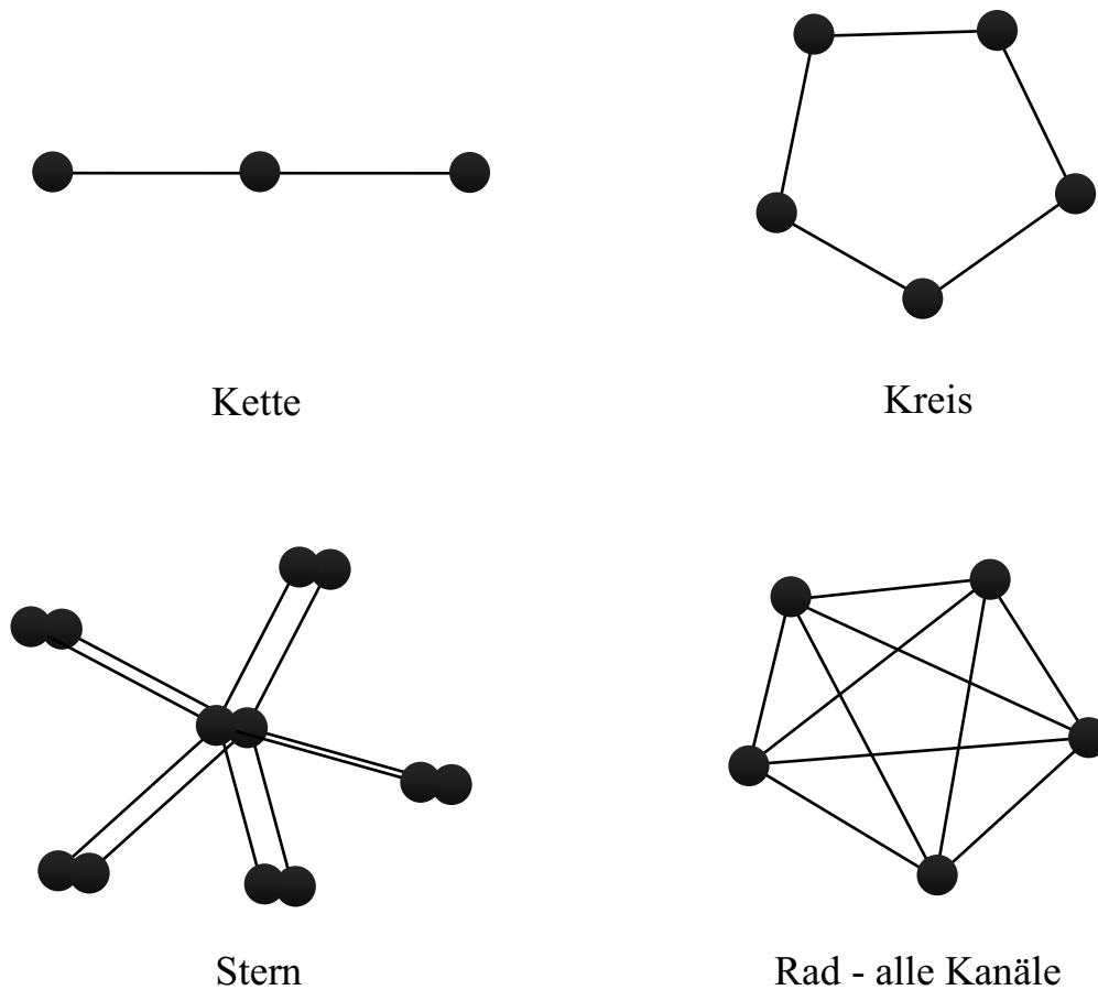
Abbildung 3: Grundformen der Kommunikation (● Kommunikationspartner, — Kommunikationsweg).
