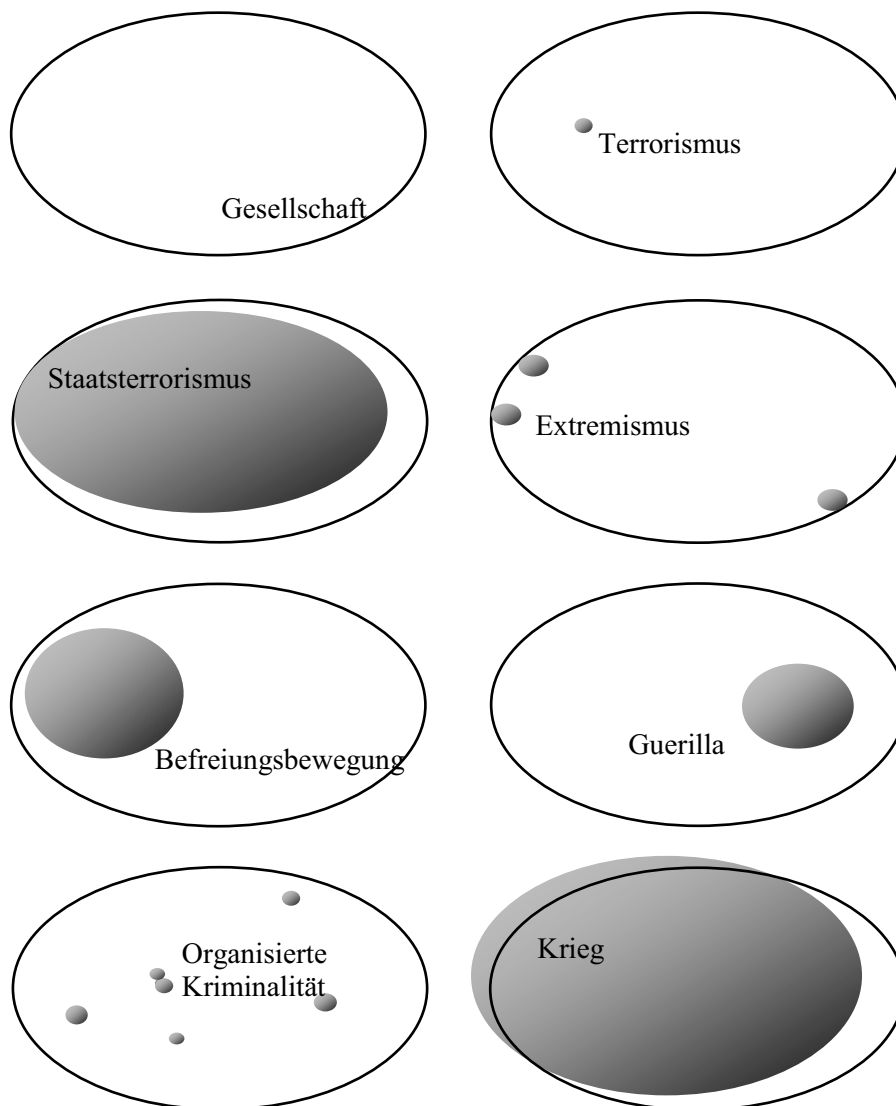
Abbildung 2: Gegenüberstellung verschiedener Gewaltformen im Verhältnis zur Gesellschaft.
