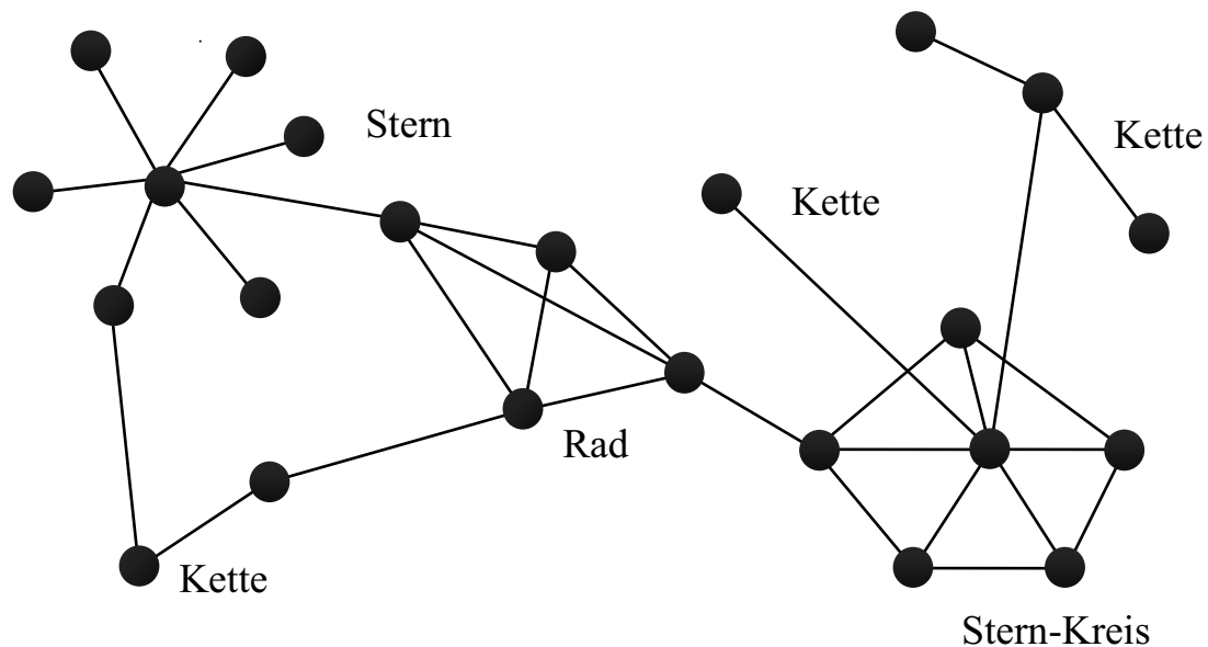
Abbildung 4: Beispielhafte Netzwerk-Kombination aus kreis-, rad-, stern- und kettenförmiger Kommunikation. Jeder Elementpunkt kann dabei ein weiteres, beliebiges Netzwerk darstellen (● Kommunikationspartner, — Kommunikationsweg).
