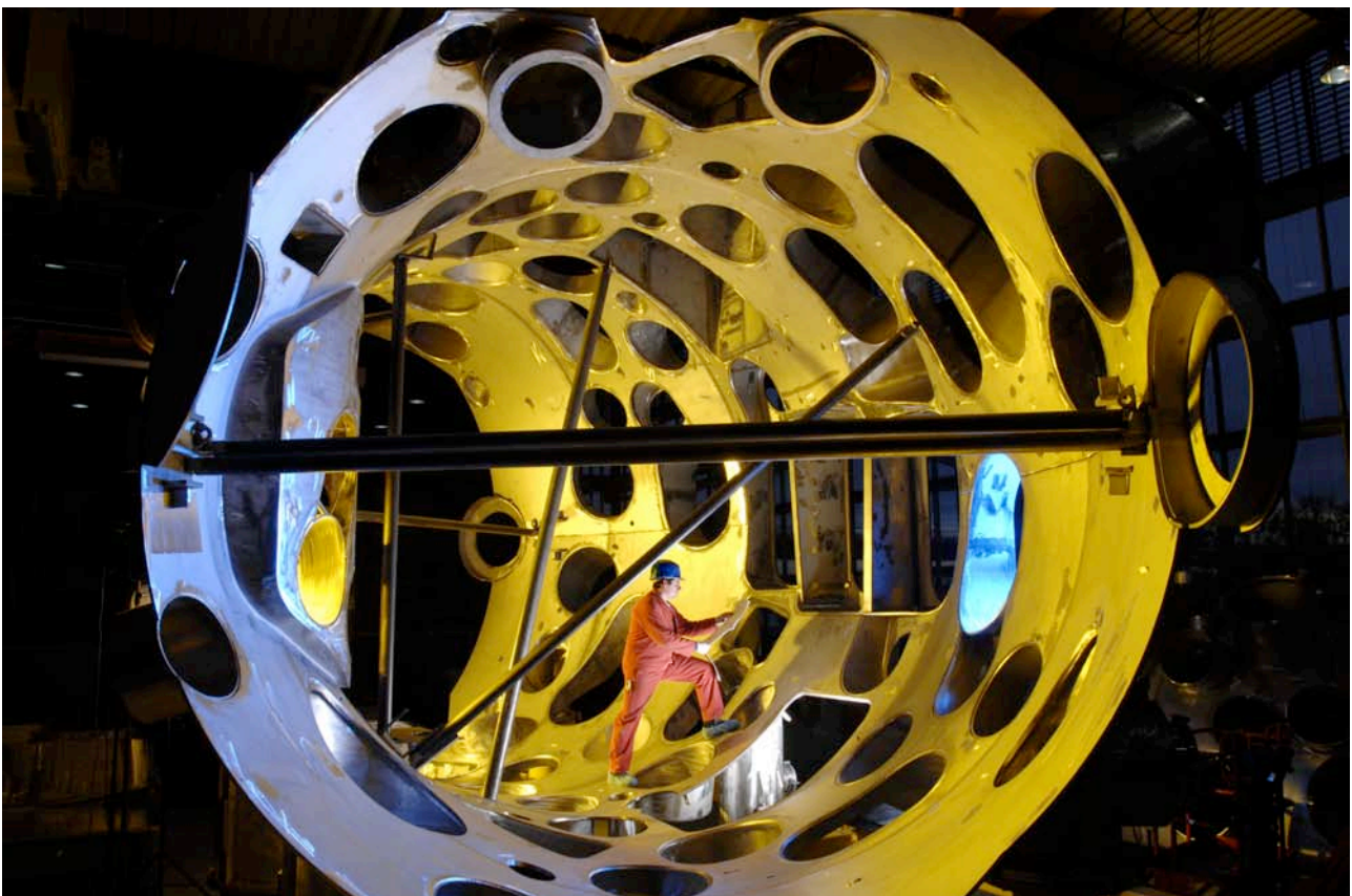
Abb. 1: Eines der fünf Teilstücke des Außengeäßes von Wendelstein 7-X (Foto: IPP, Wolfgang Filser)
