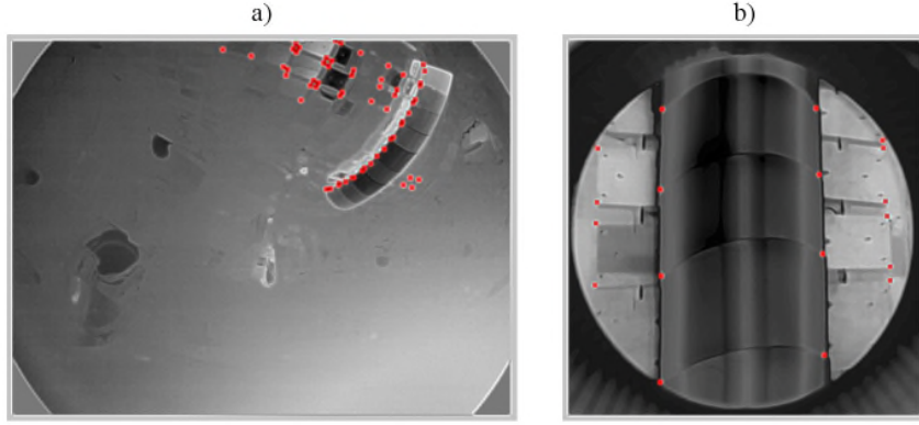
FIG. 5 Calibration points a) LWIR b) MWIR
