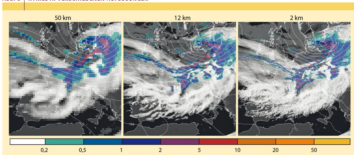
Schnappschuss vom Sturm Kyrill in Modellen mit verschiedenen Auflösungen. Weiß: Wolken, Farbschattierung: Niederschlag in mm h -1 (aus [19]).
