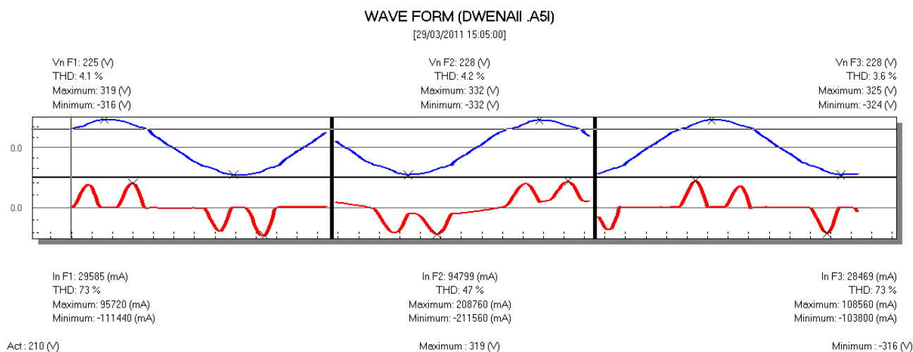
Рис. 6. Графики форм напряжения и тока
