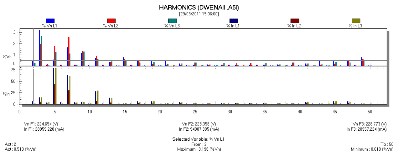
Рис. 7. График значений гармоник тока и напряжения
