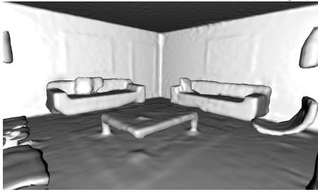
Mixture (Ours)
