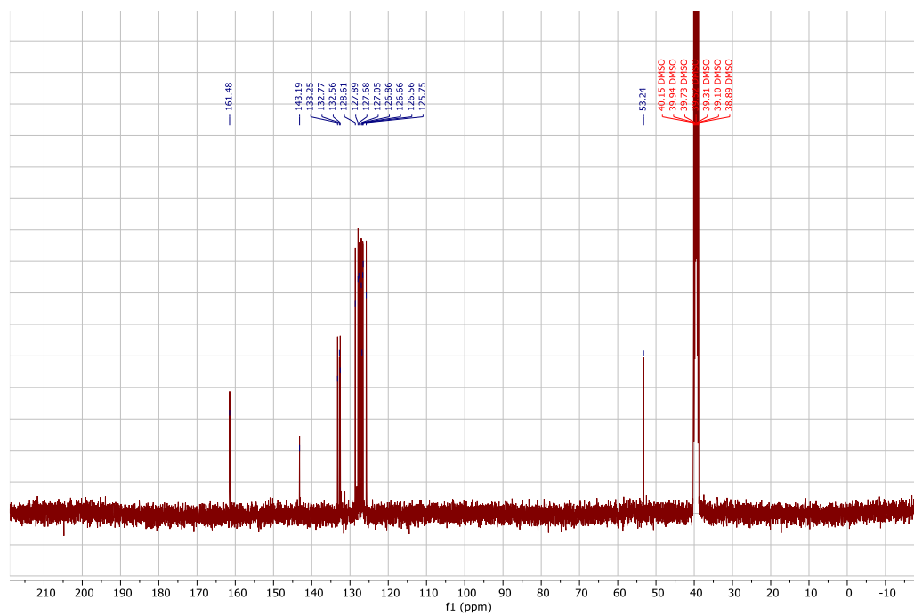
Figure 6.12. 13 C NMR 13
