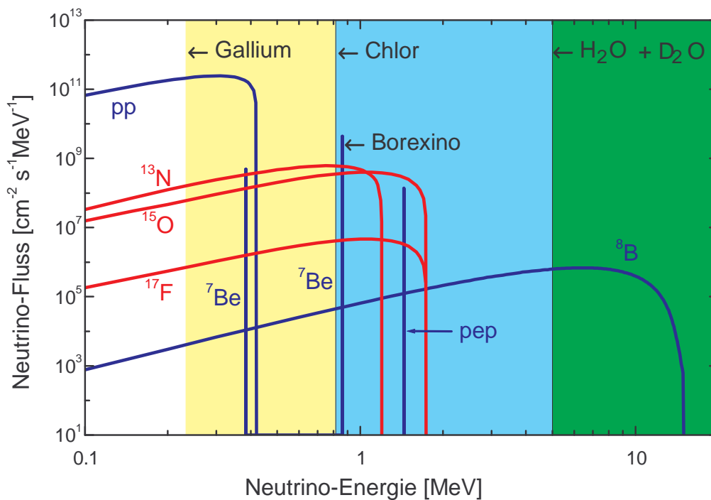
Energiespektrum der Sonnenneutrinos aus dem pp-Zyklus (blau) bzw. dem CNO-Zyklus (rot) auf der Erde nach dem Standard-Sonnen-Modell [4]. Die verschiedenen Detektoren (Ga, Cl, H 2 O, D 2 O und Borexino) detektieren Sonnenneutrinos ab der jeweils eingezeichneten Energie-Schwelle (siehe Text).
